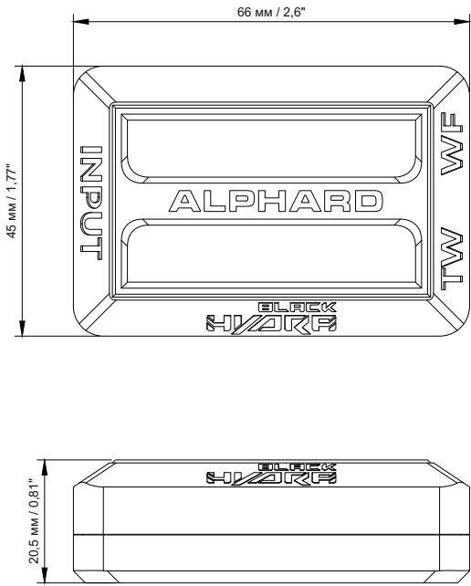
Кроссовер DELTA 613C
