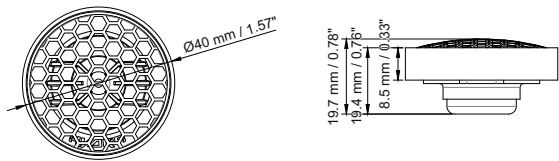
Tweeter DELTA 613C
